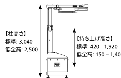
運転時(作業中)の最高高さ [mm]
