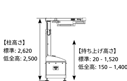
運転時(作業中)の最低高さ [mm]
