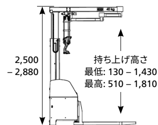
ピッキング作業中のクレーン柱高さ と持ち上げ高さ [mm]
