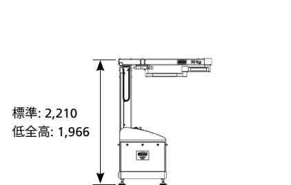
フォークリフトで移動中(作業停止時)の クレーン柱高さ [mm]
