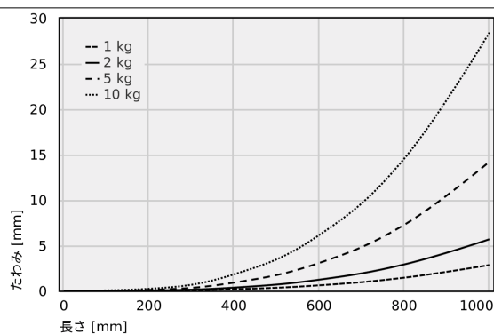
たわみパイプ 25 x 5 mm
