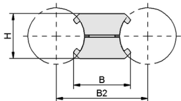
デザインデータ VBR-PR 38x30x24 P
