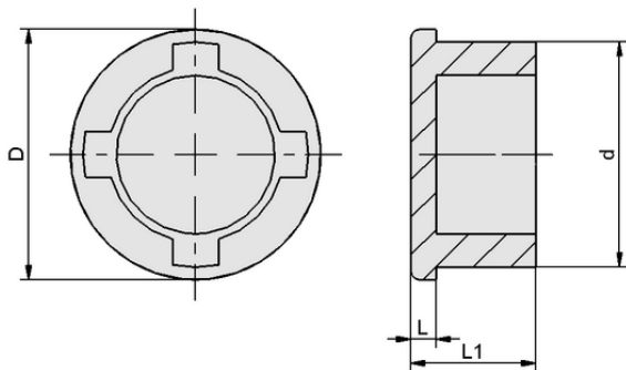
Datos de diseño KAPP 30x3 PXT D30-I
