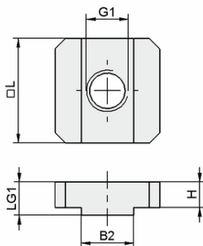
Dati di costruzione NUT-STEI 20x20 M6-IG 10
