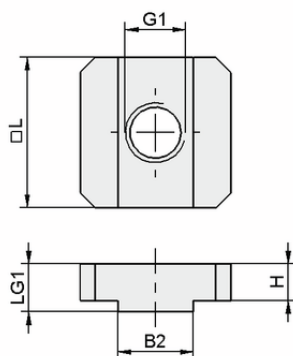
Données de construction NUT-STEI 20x20 M6-IG 10
