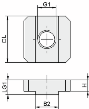
デザインデータ NUT-STEI 20x20 M6-IG 10
