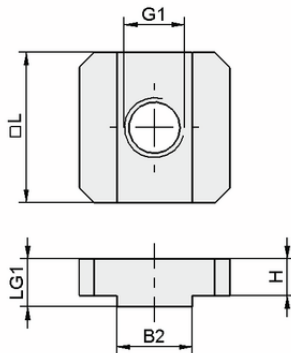
Datos de diseño NUT-STEI 20x20 M6-IG 10
