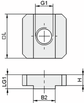
Tasarım verileri NUT-STEI 20x20 M6-IG 10
