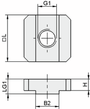
Tasarım verileri NUT-STEI 20x20 M8-IG 10
