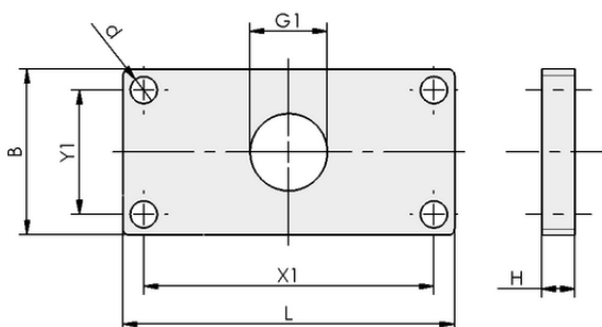
デザインデータ VRS-PL-80x40 G1/2-IG MO-PROF
