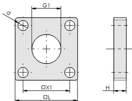
デザインデータ VRS-PL-40 G1/2-IG MO-PROF
