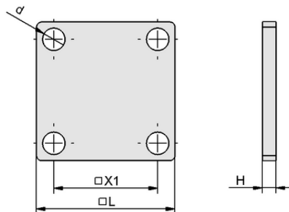
Konstruktionsdaten VRS-PL-40 MO-PROF
