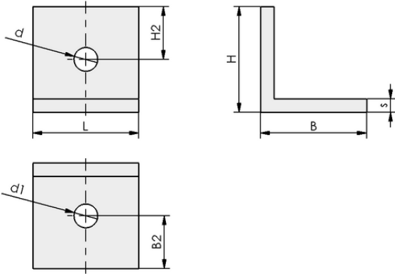
Tasarım verileri BEF-WIN 40x40x40 5 MO-PROF
