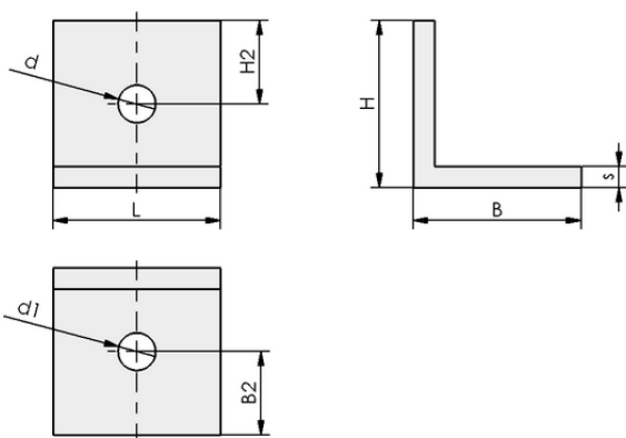
Konstruktionsdaten BEF-WIN 40x40x40 5 MO-PROF
