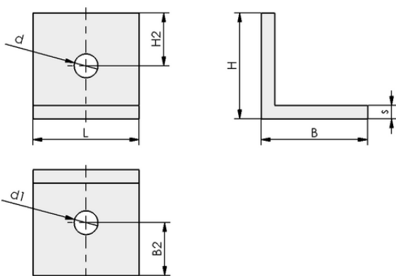
Datos de diseño BEF-WIN 40x40x40 5 MO-PROF
