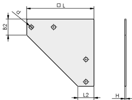
デザインデータ VBR-PR 150x3 E-FL
