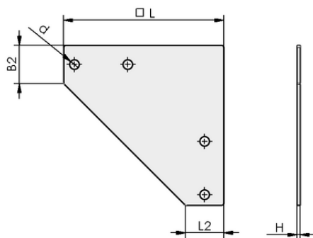
Konstruktionsdaten VBR-PR 150x3 E-FL
