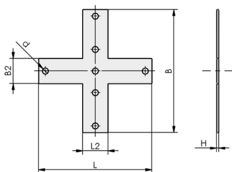
デザインデータ VBR-PR 185x185x3 K-FL
