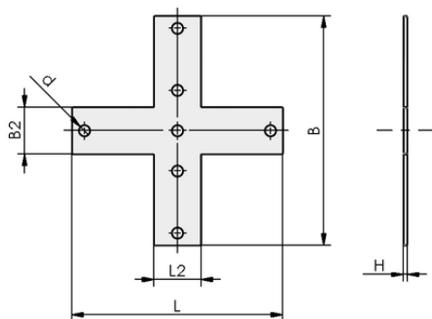
Datos de diseño VBR-PR 185x185x3 K-FL
