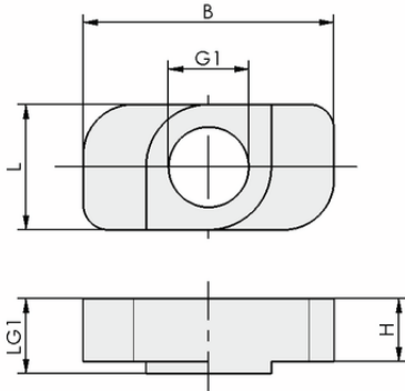
Tasarım verileri NUT-STEI 10x20 M8-IG
