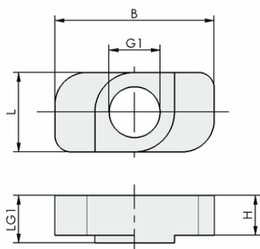
デザインデータ NUT-STEI 10x20 M8-IG
