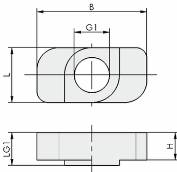
Datos de diseño NUT-STEI 10x20 M8-IG
