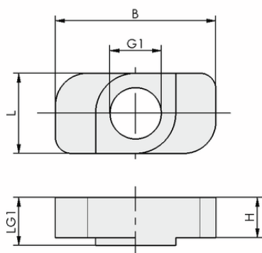
Конструктивные данные NUT-STEI 10x20 M6-IG
