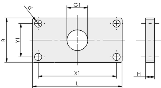
Konstruktionsdaten VRS-PL-80x40 MO-PROF
