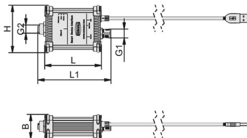
Konstruktionsdaten SDI IOL M12-5 24V-DC 24V-DC
