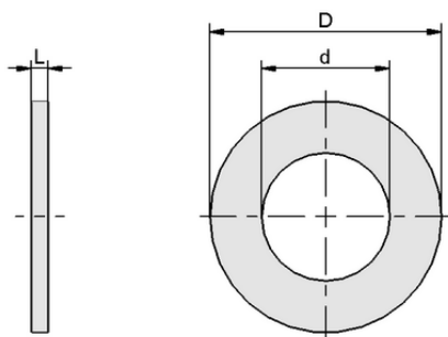
Données de construction SCHE 7090 M30 ST-HV VZ
