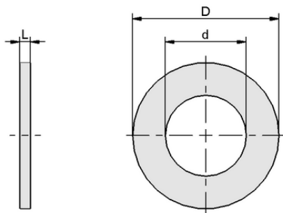
Design data SCHE 7090 M30 ST-HV VZ
