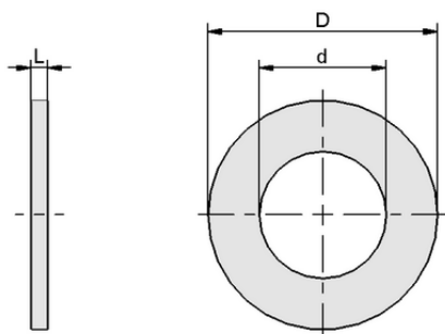
Konstruktionsdaten SCHE 7090 M30 ST-HV VZ
