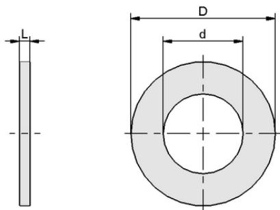
Datos de diseño SCHE 7090 M30 ST-HV VZ
