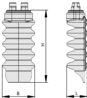
Datos de diseño FINGER-SPARE-UNIT 3CA
