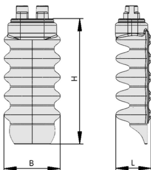
デザインデータ FINGER-SPARE-UNIT 6C
