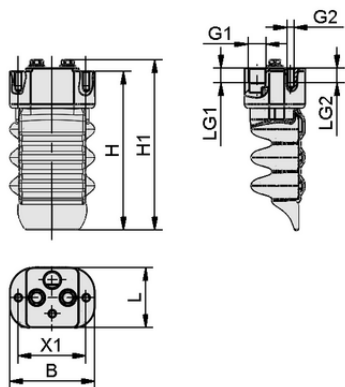
Datos de diseño FINGER-MODULE-3CA-B-AL-SI
