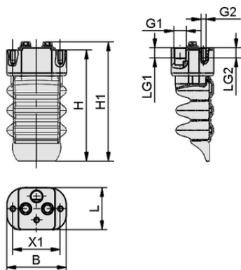
Datos de diseño FINGER-MODULE-6C-B-AL-SI
