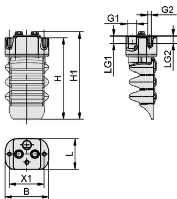
Données de construction FINGER-MODULE-5C-B-AL-SI
