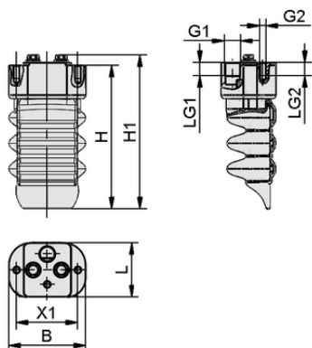
デザインデータ FINGER-MODULE-4C-B-AL-SI
