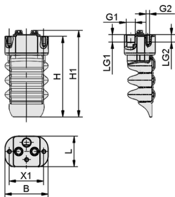
Datos de diseño FINGER-MODULE-3C-B-AL-SI
