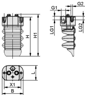
Datos de diseño FINGER-MODULE-2C-B-AL-SI
