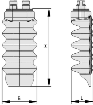
Tasarım verileri FINGER-SPARE-UNIT 6C IND
