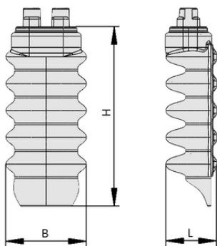
Datos de diseño FINGER-SPARE-UNIT 5C IND
