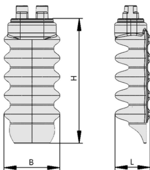
Datos de diseño FINGER-SPARE-UNIT 3CV IND
