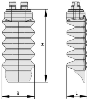
Données de construction FINGER-SPARE-UNIT 3CA IND
