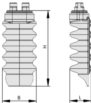
Datos de diseño FINGER-SPARE-UNIT 2C IND
