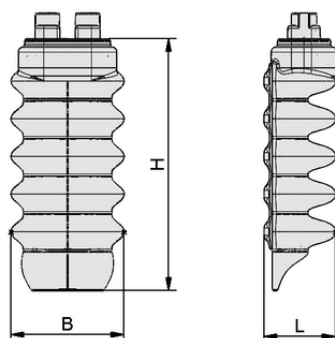
Données de construction FINGER-SPARE-UNIT 6C HYG
