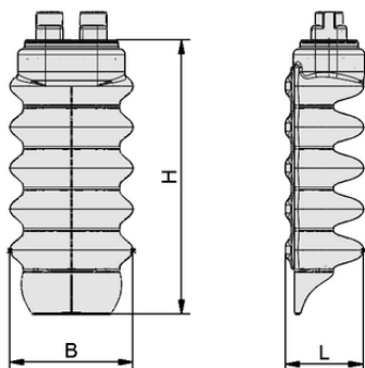
Datos de diseño FINGER-SPARE-UNIT 5C HYG
