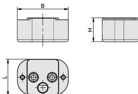
Datos de diseño FINGER-COMP BASE A4 HYG
