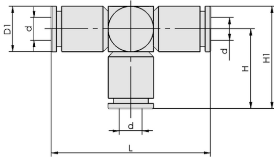
Tasarım verileri SVB-T 14
