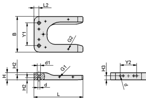
Dati di costruzione STATION 150x110x22 MATCH
