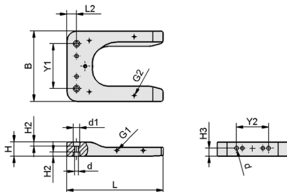
Конструктивные данные STATION 150x110x22 MATCH
