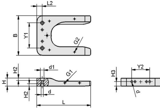
Tasarım verileri STATION 150x110x22 MATCH
